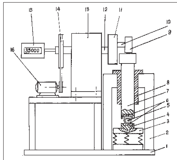
Рис. Схема стенда для дослідження цементних зразків при циклічному стиску. 1 – станина, 2 – рама, 3 – динамометр ДОСМ-3-0,1, 4 – опора, 5 – зразок, 6 – свинцеві вкладки, 7 – штовхач, 8 – втулка, 9 – підшипник, 10 – палець, 11 – ексцентрик, 12 – вал, 13 – корпус, 14 – клиноремінна передача, 15 – лічильник кількості обертів СКО –1, 16 – електродвигун АОЛ –012/14.
